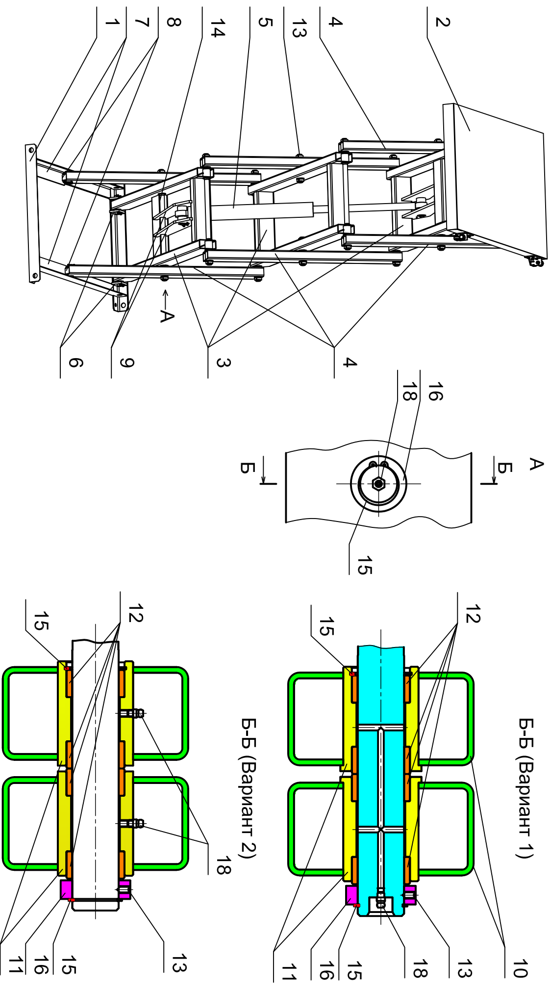
Рис. 1. Стол подвёмный ножничный
